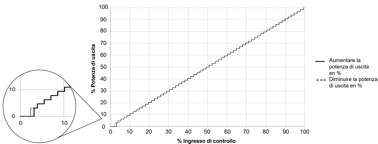
Modalità di commutazione a 4 cicli completi: RGC...C4
