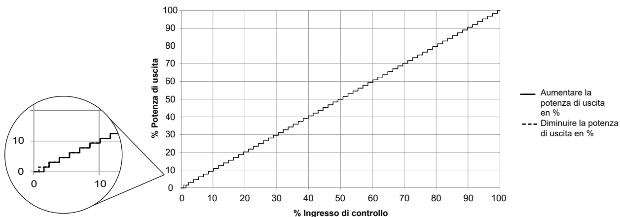
Modalità di commutazione a 1 ciclo completo: RGC...C1
