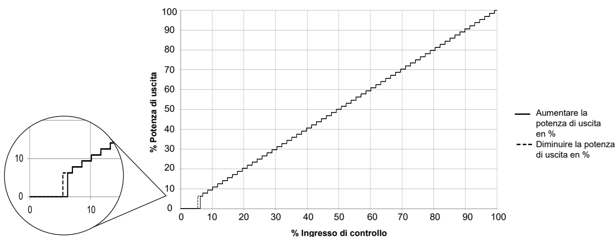
Modalità di commutazione a 16 cicli completi: RGC...C16
