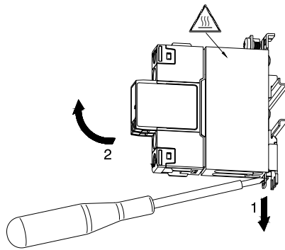
Smontaggio della guida DIN
